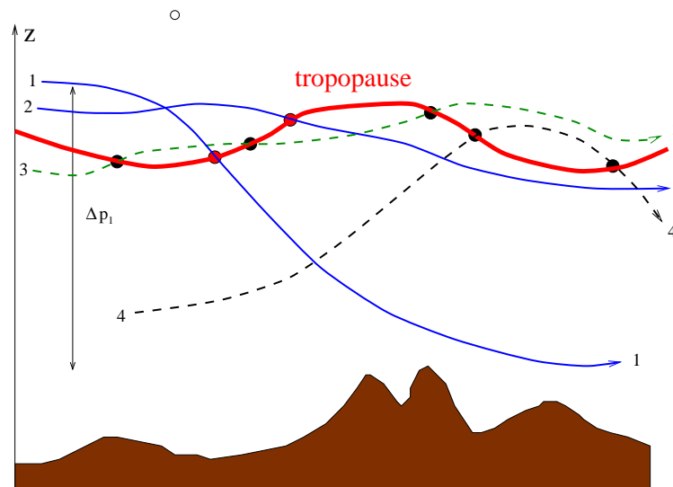
Fig. 11 Schematische Darstellung zum Stratosphären-Troposphären Austausch: Alle eingezeichneten Trajektorien durchstossen die Tropopause, jedoch nur bei den Trajektorien 1 und 2 ist der Austausch bedeutsam, d.h. von einer gewissen zeitlichen Dauer. Die Trajektorie 3 hingegen pendelt ständig zwischen der Tropo- und der Stratosphäre hin und her, und die Trajektorie 4 ist nur für eine sehr kurze Zeit in der Stratosphäre bevor sie wieder in die Troposphäre zurückkehrt. Bei der Trajektorie 1 ist die Vertikalbewegung \Delta p gross, sie stellt ein sogenanntes “tiefes Austauschereignis” dar.
