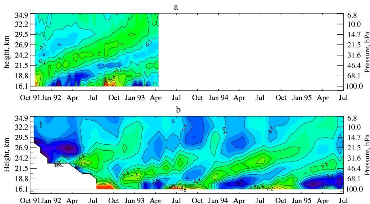
Fig. 24 Höhe/Zeit-Querschnitte des (a) MLS Mischungsverhältnis q von Wasserdampf, dargestellt als Abweichung vom zeitgemittelten Profil zwischen 12S und 12N und (b) HALOE \hat{H} = 2(\text{CH}_4) + (\text{H}_2\text{O}) , des variablen Wasseranteils zwischen 12S und 12N [entnommen aus „An atmospheric tape recorder: The imprint of tropical tropopause temperature on stratospheric water vapor“, P. W. Mote et al., J. Geophys. Res. , Vol. 101 (D12), 3989-4006, February, 1996].
