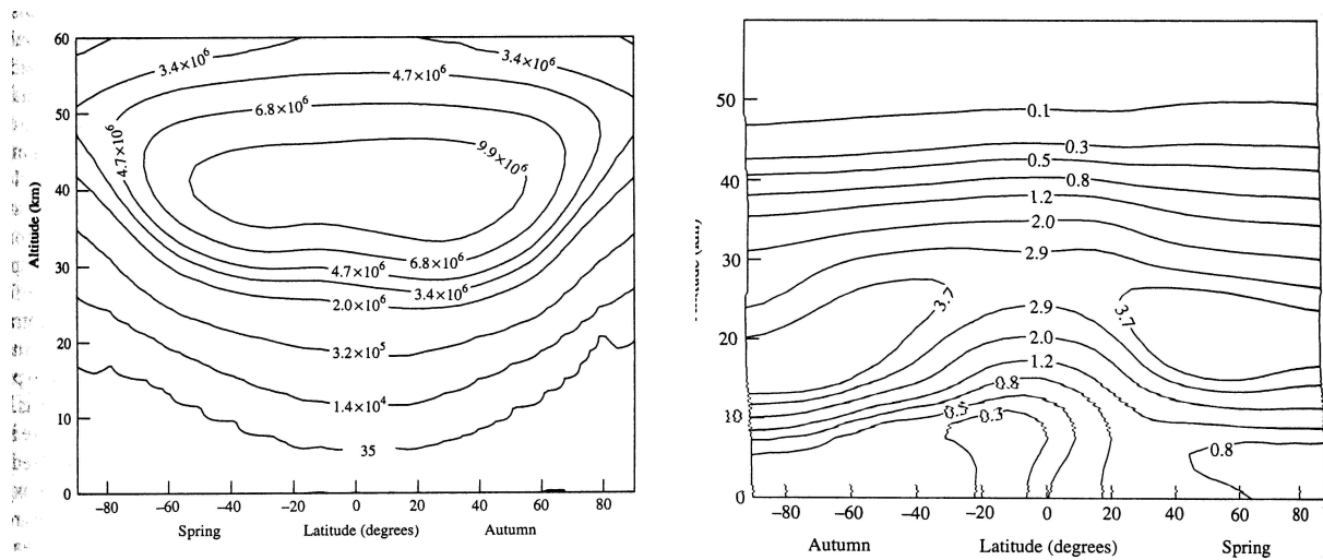
Fig. 19 Links: Zonal gemittelte Rate der Ozonbildung durch Photolyse von O_2 in Einheiten von Moleküle cm^{-3} s^{-1} . Rechts: Zonal gemittelte Ozonkonzentration in 10^{12} Moleküle cm^{-3} als Funktion von Höhe und Breite. [Berechnet von D. E. Shallcross, abgebildet in „Chemistry of Atmospheres“, R. P. Wayne].
