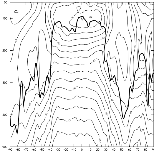
Fig. 22 Temperatur (in Grad Celsius) und 2 pVU/380 K-Tropopause in einem Nord/Südschnitt. Beachte, dass die tiefsten Temperaturen bei der tropischen Tropopause auftreten. Sie beträgt hier ca. -70 Grad Celsius, während in den Ausertropen typischerweise -50 Grad Celsius beobachtet werden.
