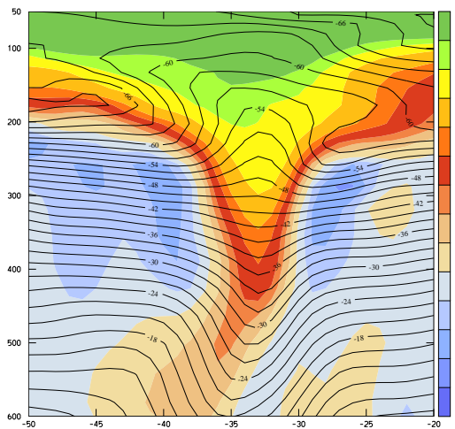
Fig. 4 PV und Temperatur in einem Ost/West-Schnitt durch einen stratosphärischen PV-Streamer. Man erkennt deutlich, dass mit dem PV-Streamer eine tiefe dynamische Tropopause einhergeht. Das Temperaturfeld wird hingegen durch den PV-Streamer so deformiert, dass das Lapse-Rate-Kriterium der thermischen Tropopause erst in grossen Höhen erreicht wird. Damit liegt hier die thermische Tropopause bedeutend höher als die dynamische Tropopause.
