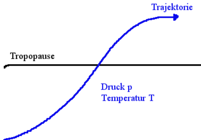
Fig. 20 Schematische Darstellung einer Trajektorie, die durch die Tropopause stösst. Für den Feuchtetransport ist massgeblich, welcher Druck und welche Temperatur beim Durchstossungspunkt durch die Tropopause vorherrscht. Diese beiden Werte legen das Sättigungsmischungsverhältnis w_s fest.
