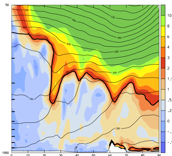
Fig. 8 Definition der dynamischen Tropopause. In den Aустertropen fällt diese mit der 2 pvu Isfläche der potentiellen Vortizität zusammen, in den Tropen mit der 380 K-Isentropen. Formal ist sie definiert durch den Druck p(\text{Tropopause}) = \max(p@2, pvu, p@380 K) . Die vertikale Skala ist in \log(p) aufgetragen, wobei die Striche links 100 hPa-Abstände markieren. Folgende Merkregel kann hilfreich sein für die Höhe der Tropopause: Tropen 100 hPa, mittlere Breiten 200 hPa, Polargebiete 300 hPa.
