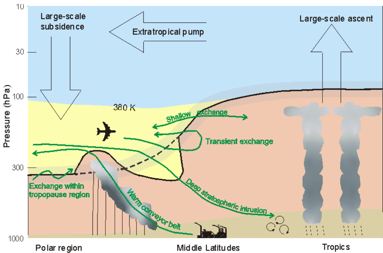
Fig. 18 Globale Perspektive des Massenaustauschs durch die Tropopause. Die mittlere Lage der Tropopause ist durch die dicke schwarze Linie gekennzeichnet. Blau ist die „Overworld“ unterlegt, in der sich die Isentropen (über 380 K) ganz in der Stratosphäre befinden. Das gelb markierte Gebiet ist die „Lowermost Stratosphere“, bei der die Isentropen die Tropopause schneiden, dh. ein Teil einer isentropen Fläche befindet sich in der Stratosphäre und ein Teil in der Troposphäre. Die freie Troposphäre ist violett dargestellt und die atmosphärische Grenzschicht braun. Die breiten Pfeile geben den Massetransport in der globalen Perspektive an, die schmalen Pfeile den Transport von Luftmassen durch die extratropische Tropopause. Die gelb markierten Auswuchtungen der Tropopause ergeben sich oft im Zusammenhang mit „Warm Conveyor Belts“ und mit tiefreichenden stratosphärischen Intrusionen [entnommen aus „Stratosphere-Troposphere exchange: A review, and what we have learned from STACCATO“, Stohl, A. et al., J. Geophys. Res. , Vol. 108 (D12), 2003.
