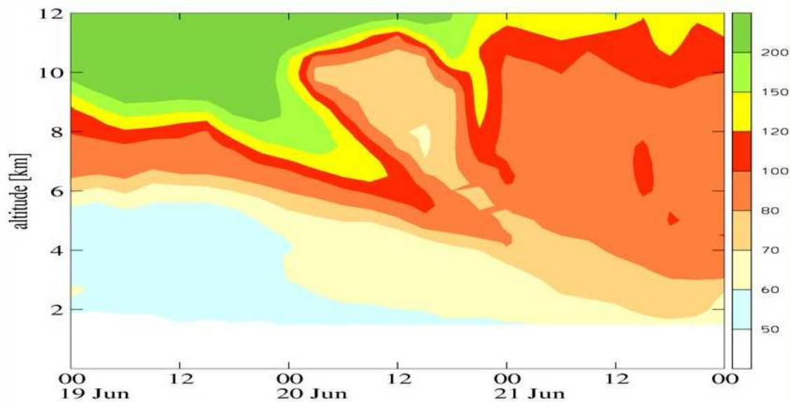
Fig. 13 Oben: LIDAR-Messungen vom 20. und 21. Juni 2001. Angegeben ist die Ozonkonzentration in ppb. Unten: Entsprechende Analyse des Ozons im ECMWF. [entnommen aus einem Vortrag von Andreas Stohl am SPARC-Workshop in Mainz, 2005].
